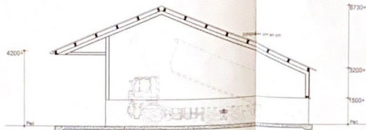
Doorsnede voeropslag/wagenberging 1:100
